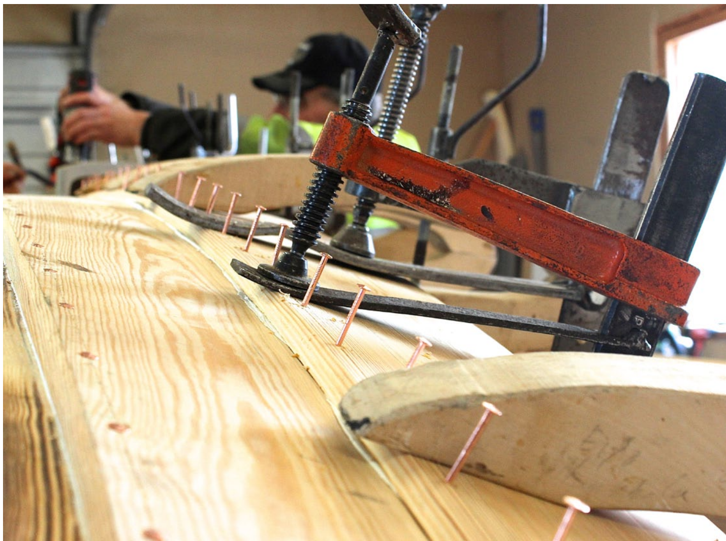
Sivulautojen kiinnittäminen puuveneeseen tapahtuu ruostumattomien kuparinaulojen, kupurikkojen ja lyöntituuran avulla.
